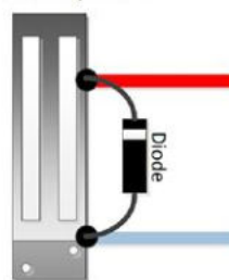
Ventouse ou gâche à rupture
